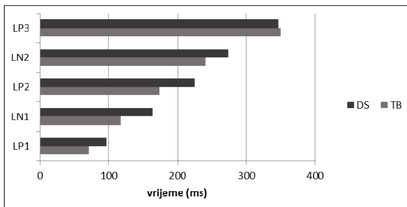
Slika 15. Grafički prikaz usporedbe latencija ciljnih podražaja TB i DS u S1
